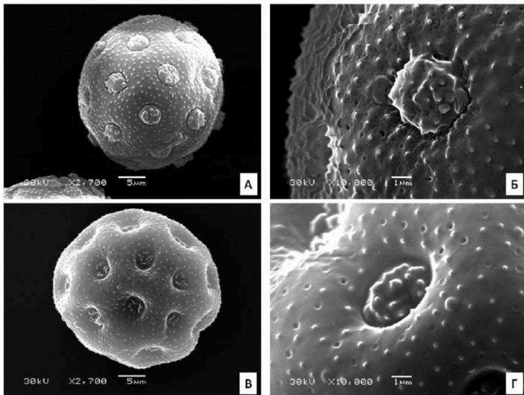
Рис. 1. Пилкові зерна A. lithuanicum (А, Б) та A. armeria (В, Г): А, Б – загальний вигляд; В, Г – пора з кришечкою
