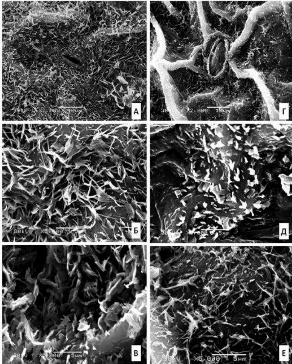
Рис. 4. Ультраскульптура листової пластинки A. lithuanicum (A-B) та A. armeria (Г-Е): А, Г – продих (Ab), Б, Д – скульптура епікутикулярного воску (Ab), В, Е – скульптура епікутикулярного воску (Ad)
